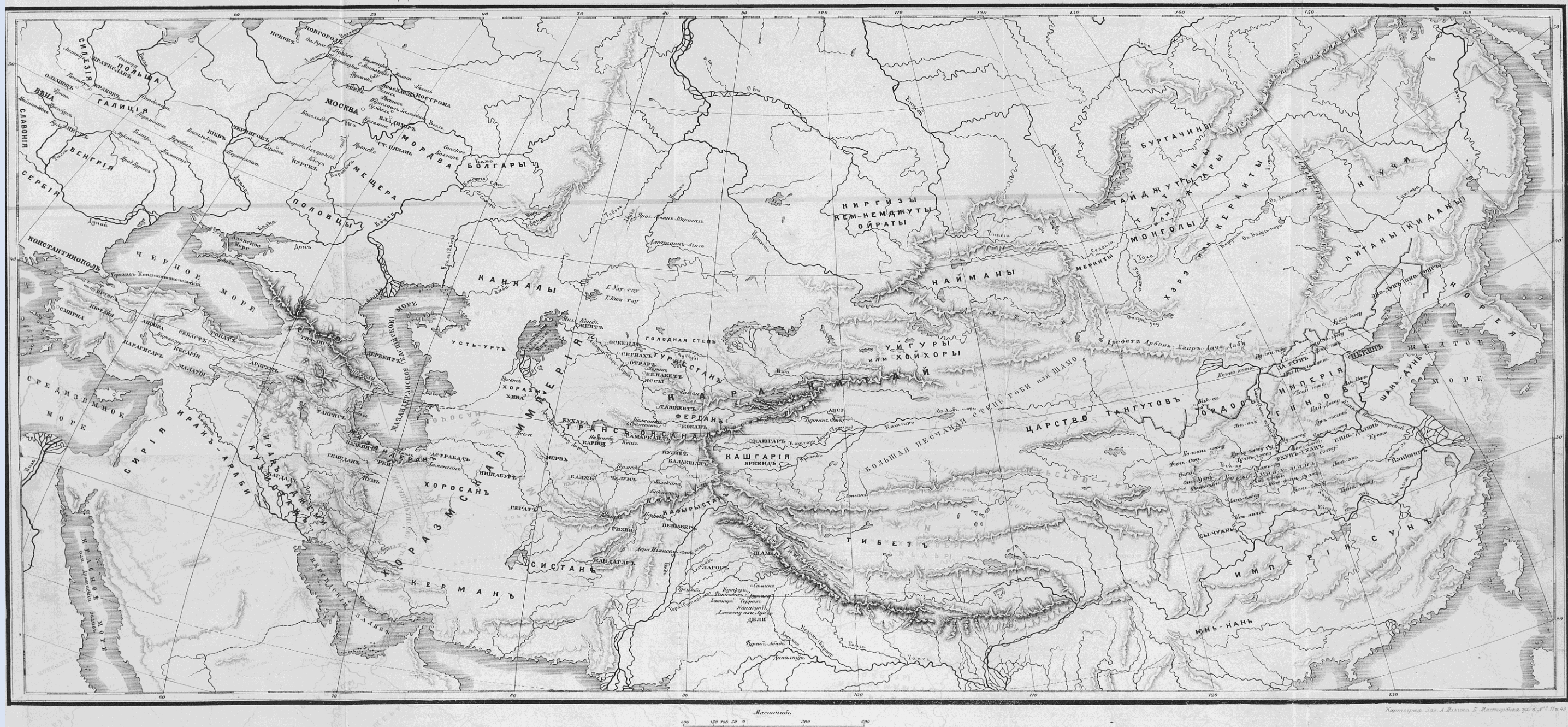
КАРТА СРЕДНЕЙ АЗИИ И ЧАСТИ ЕВРОПЫ, ДЛЯ ОБЪЯСНЕНИЯ ПОХОДОВ ЧИНГИЗЬ-ХАНА И ТАМЕРЛАНА ВЪ XIII И XIV ВѢКАХЪ.
